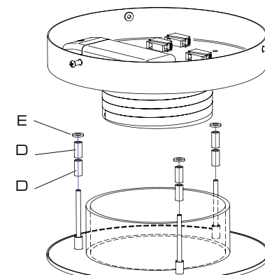
Quitar separadores D y E Remove separators D and E
